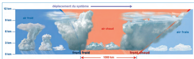
Soulèvement frontal
