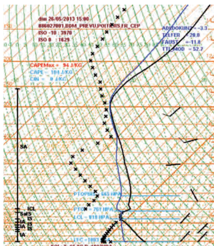
Inversion de subsidence qui limite le plafond (Cu ou thermic pur)
