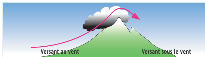
Soulèvement orographique
